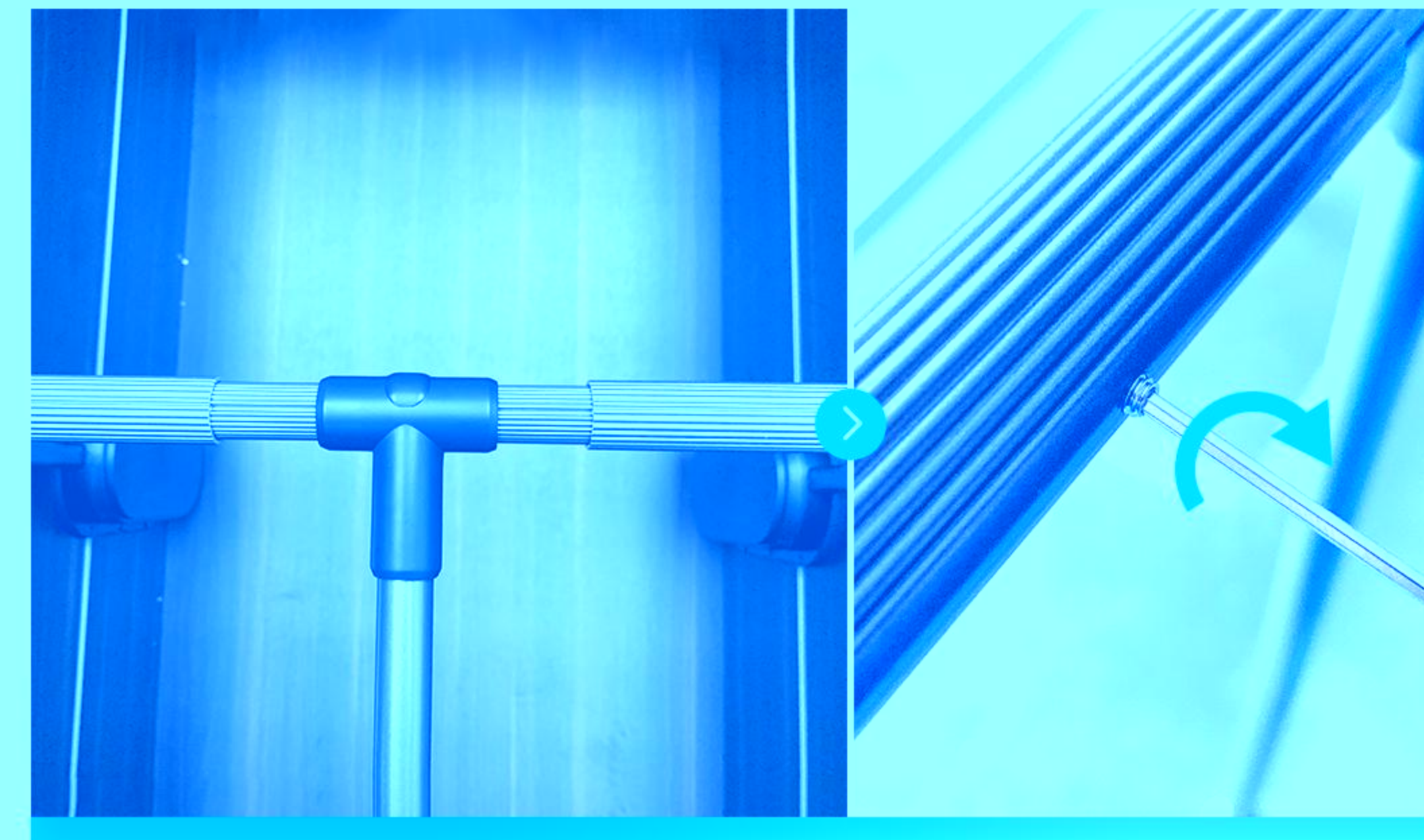
依柜子宽度， 调节好可调管并锁紧机米螺丝2个
